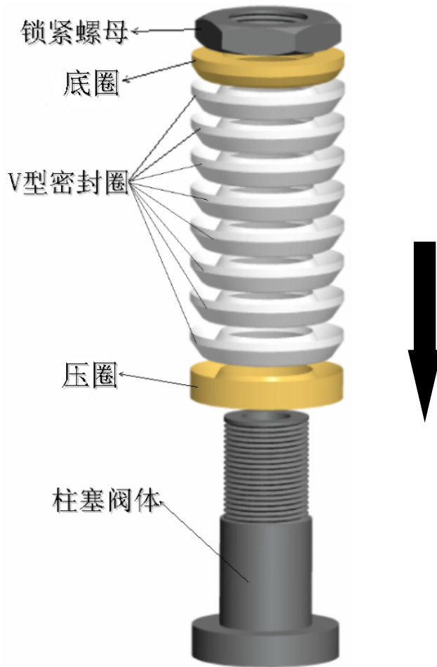
图五 柱塞阀体装配示意图
