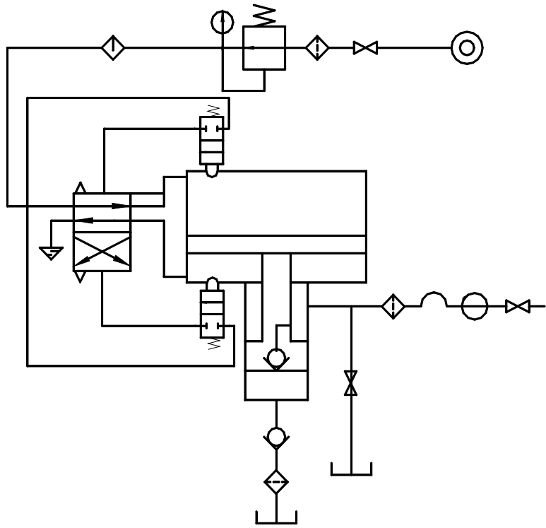
图二 QPT7037K 工作原理图
